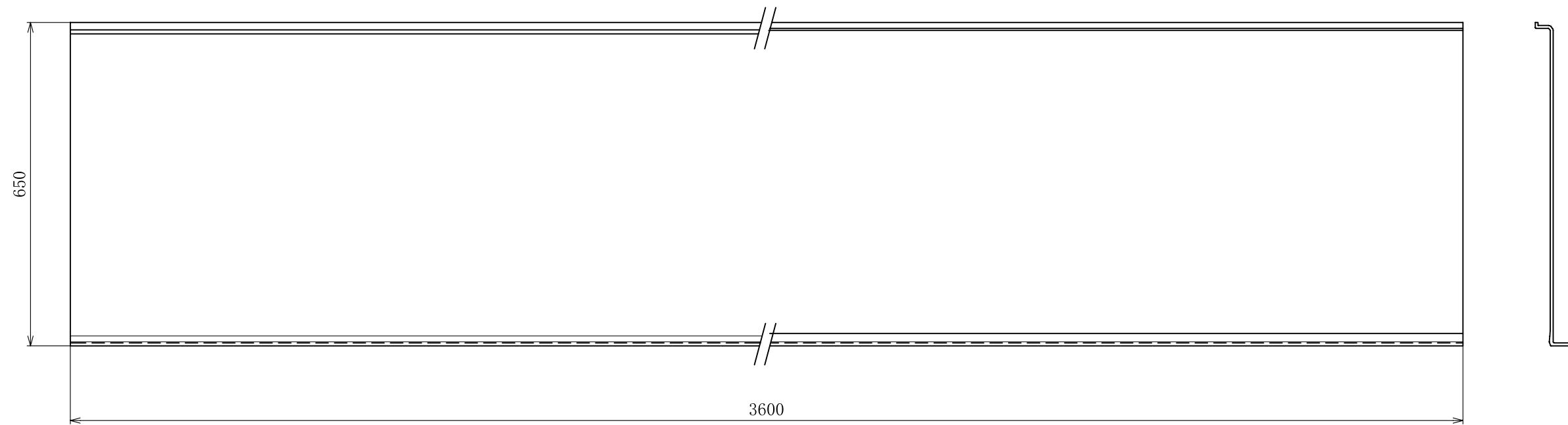
平面図 S = (1/10)
